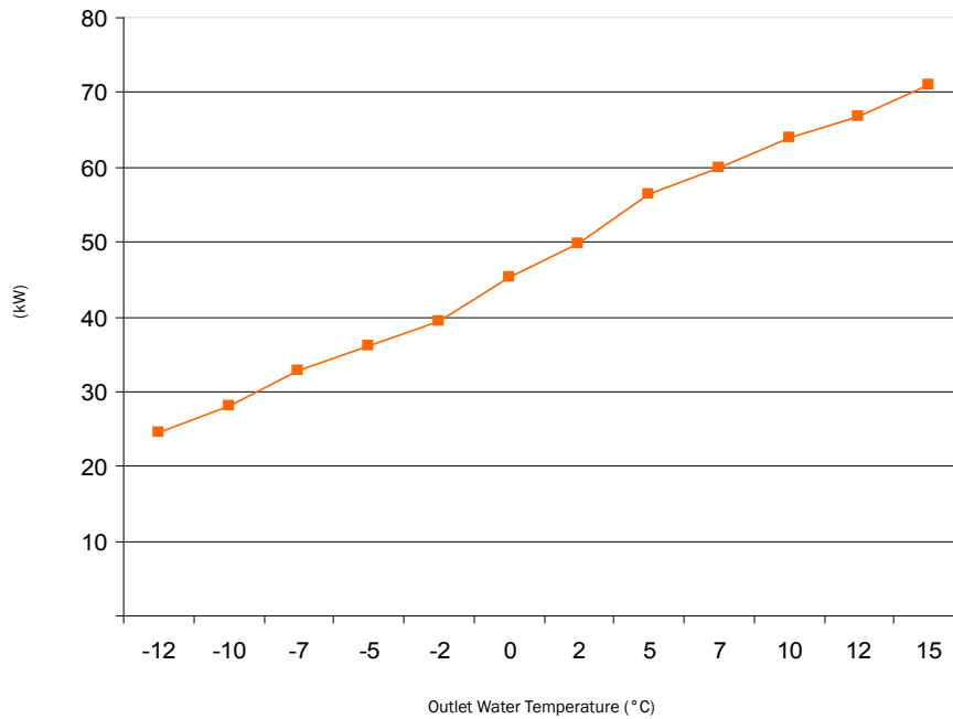
50kW LT Fan Coil
